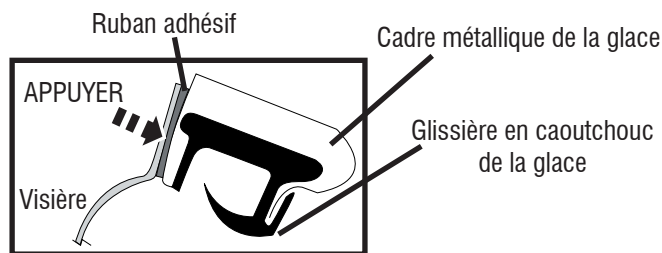
Coupe transversale de la visière en place
