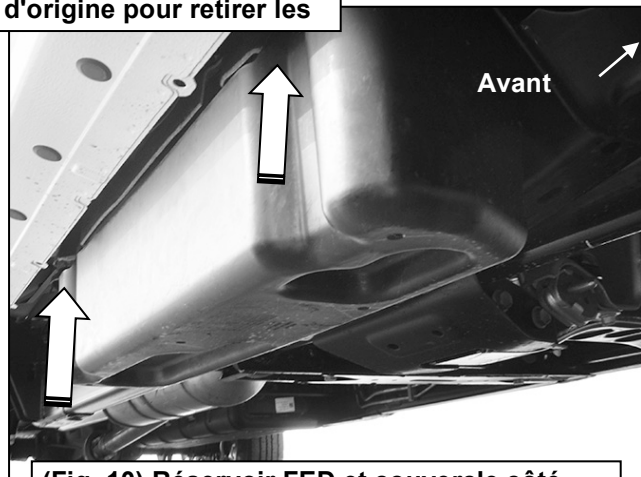
(Fig. 10) Réservoir FED et couvercle côté passager
