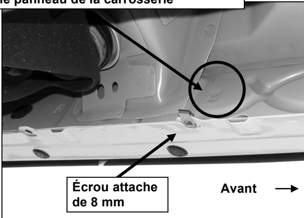
(Fig. 3) 2 ème emplacement de montage côté conducteur
