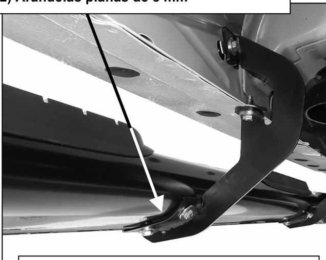
(Fig. 17) Ilustración de la instalación del lado del pasajero
