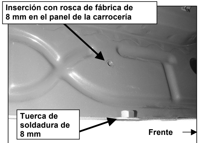
(Fig. 2) Soporte de montaje del tubo del lado del pasajero
