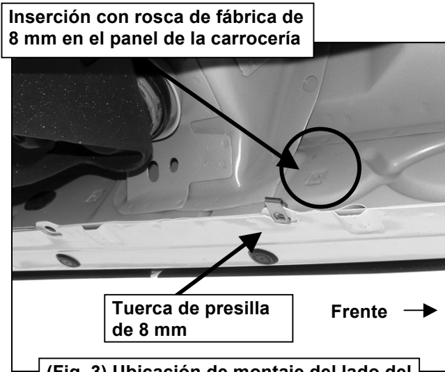
(Fig. 3) Ubicación de montaje del lado del conductor (2)
