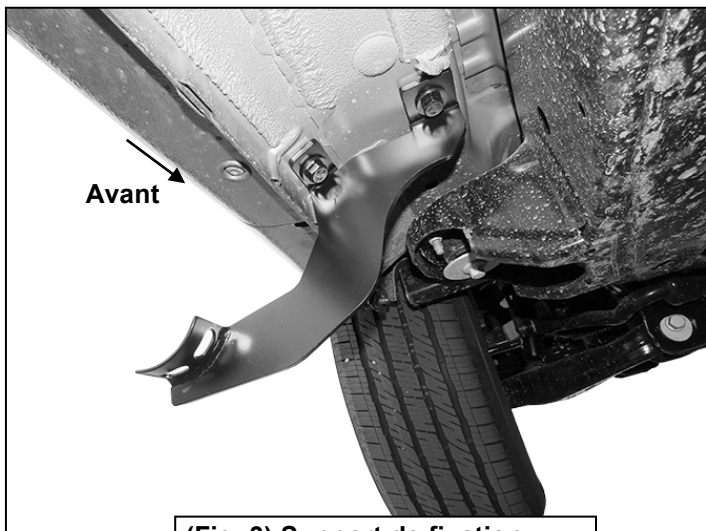
(Fig. 3) Support de fixation côté conducteur/gauche monté
