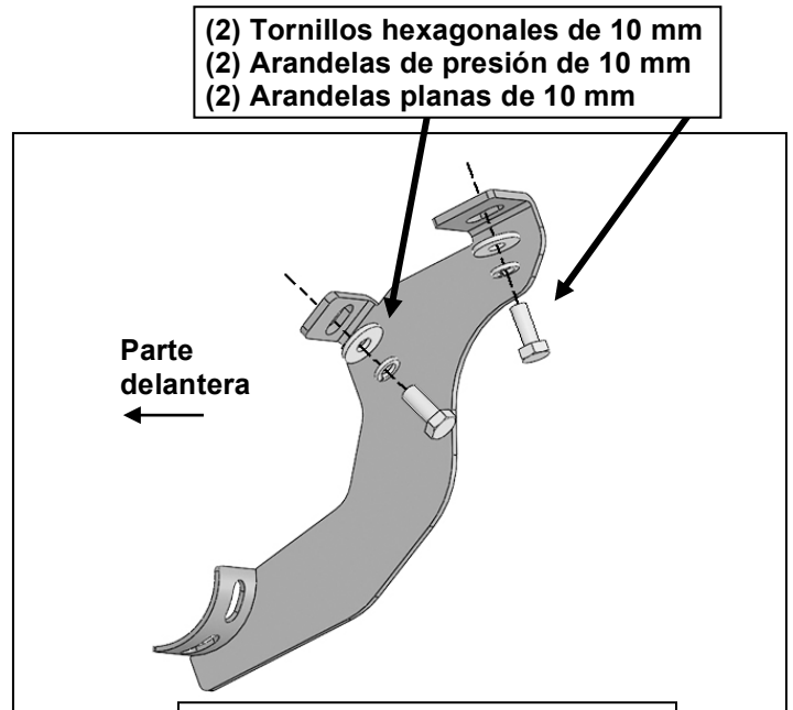
(Fig. 2) Instalación del soporte de montaje frontal izquierdo/del lado del conductor
