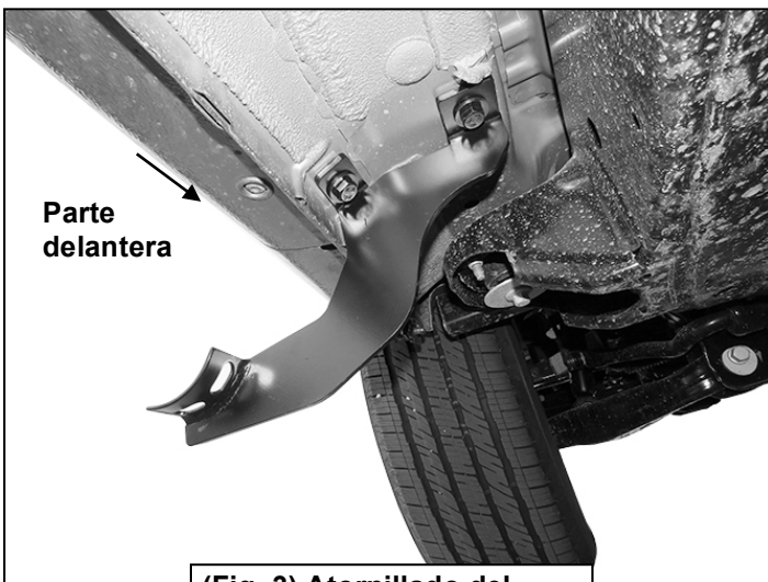
(Fig. 3) Atornillado del soporte de montaje frontal izquierdo/del lado del conductor
