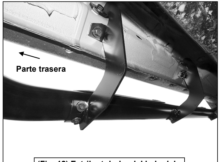
(Fig. 12) Estribo tubular del lado del conductor/izquierdo instalado al soporte de montaje trasero
