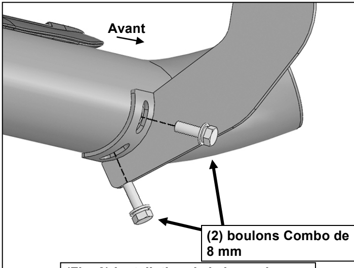
(Fig. 9) Installation de la barre de protection côté conducteur/gauche
