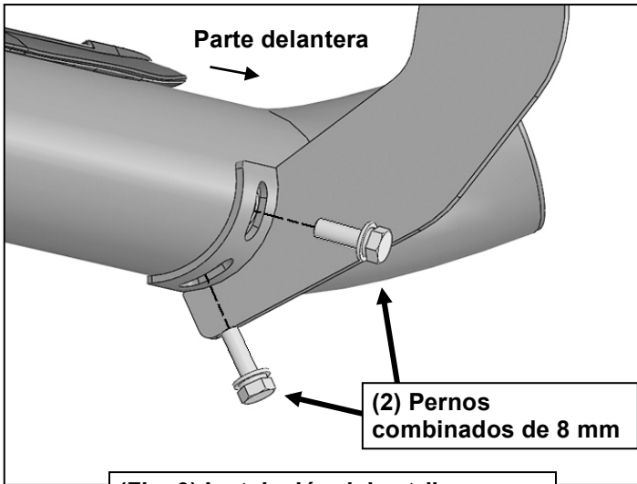
(Fig. 9) Instalación del estribo tubular izquierdo/del lado del conductor
