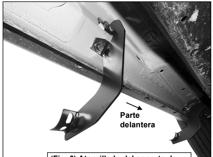
(Fig. 6) Atornillado del soporte de montaje central izquierdo/del lado del conductor
