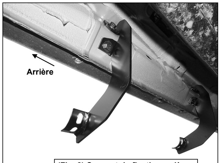
(Fig. 8) Support de fixation arrière côté conducteur/gauche installé
