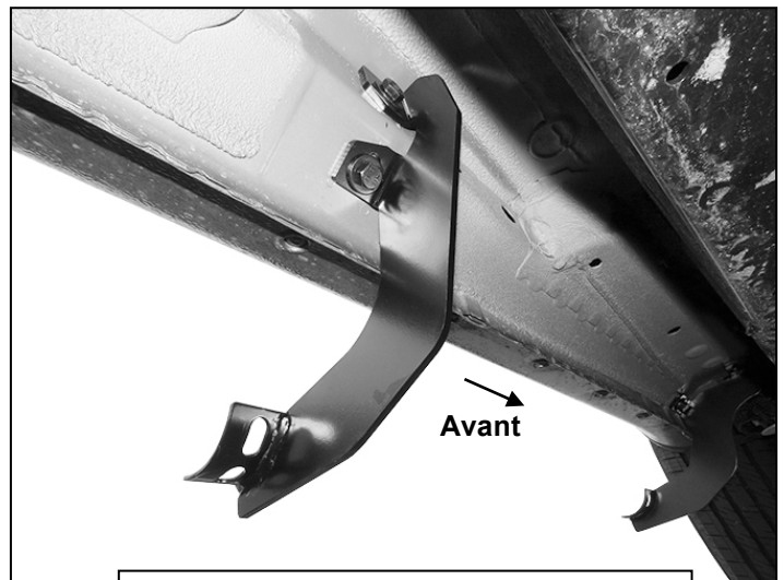
(Fig. 6) Support de fixation central côté conducteur/gauche installé
