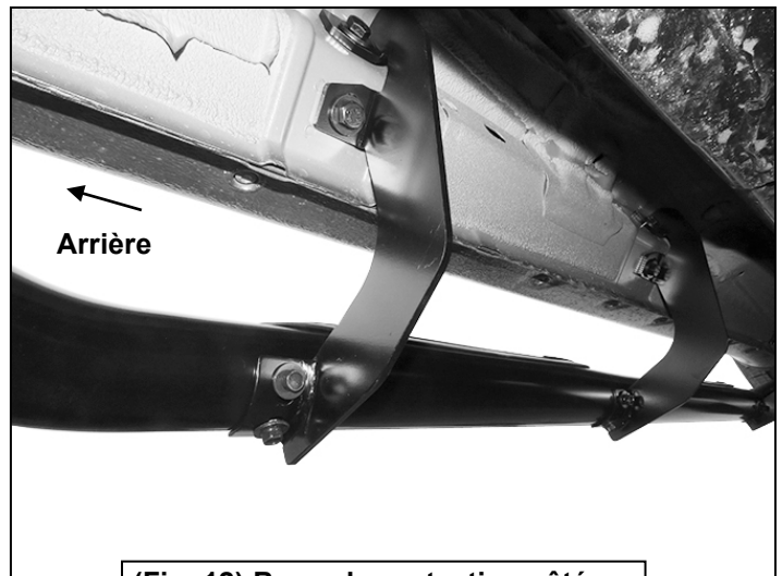
(Fig. 12) Barre de protection côté conducteur/gauche installée sur le support de fixation arrière
