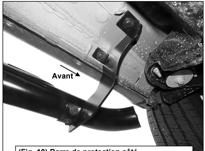
(Fig. 10) Barre de protection côté conducteur/gauche installée sur le support de fixation avant
