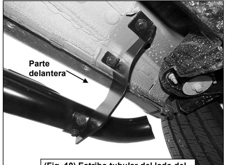
(Fig. 10) Estribo tubular del lado del conductor/izquierdo instalado al soporte de montaje frontal
