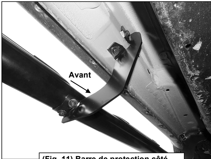
(Fig. 11) Barre de protection côté conducteur/gauche installée sur le support de fixation central
