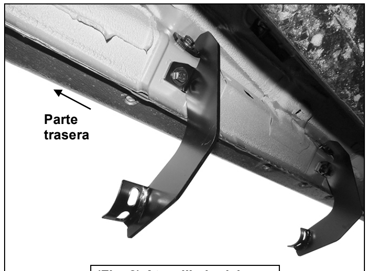
(Fig. 8) Atornillado del soporte de montaje trasero
